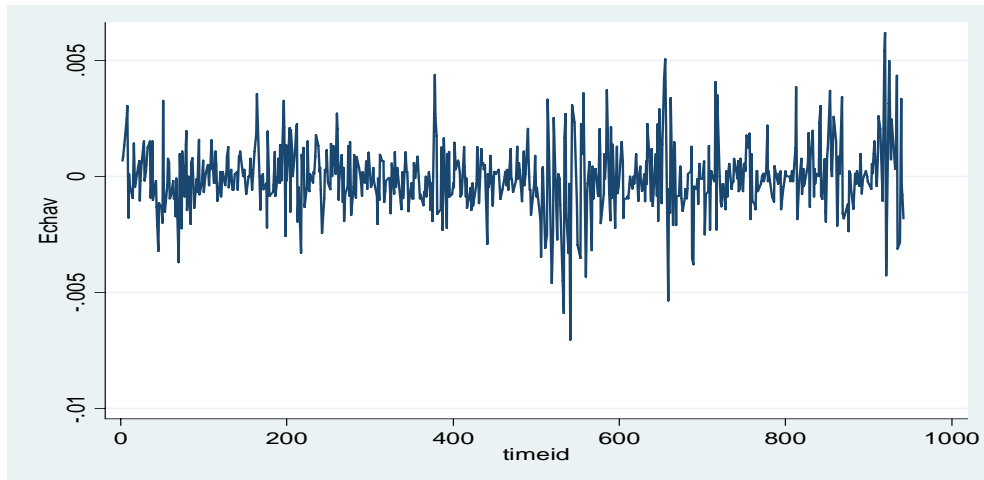
echav
